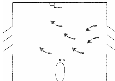
Slika 2. Postavljanje detektorske sonde za kontrolu gasova težih od vazduha. Kontrolisani prostorje bez prirodne i prinudne ventilacije.
